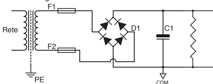
Fig.xxx : Circuito di alimentazione dello stadio di potenza
