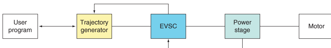
Fig.xxx : Schema della catena di controllo in open loop
