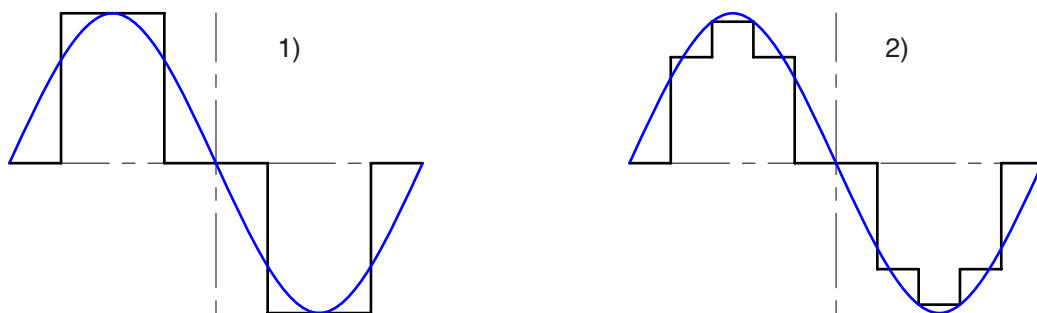
Fig.xxx : Differenza di profilo di corrente tra un azionamento tradizionale e i drive VectorStep a passo intero (1) e a mezzo passo (2)
