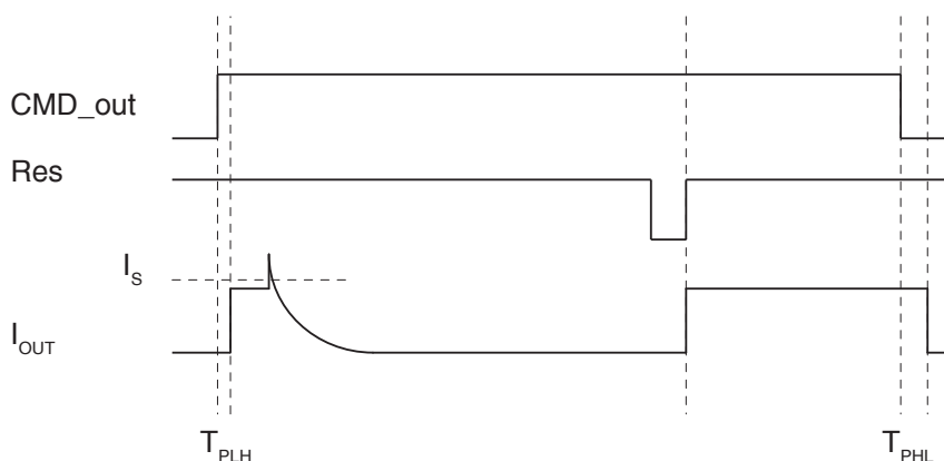
Fig.xxx : Comportamento di un'uscita in caso di sovraccarico
