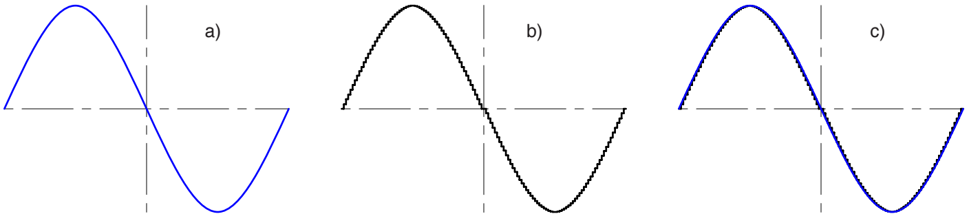
Fig.xxx : Profilo di corrente al motore: a) VectorStep con tecnologia stepless b) azionamento microstep tradizionale c) confronto dei profili
