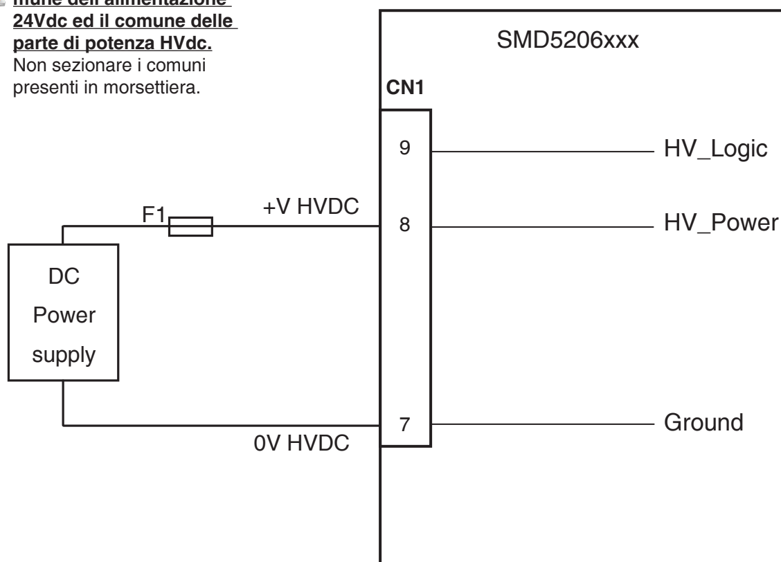
Fig.xxx : Circuito di alimentazione dello stadio di potenza
