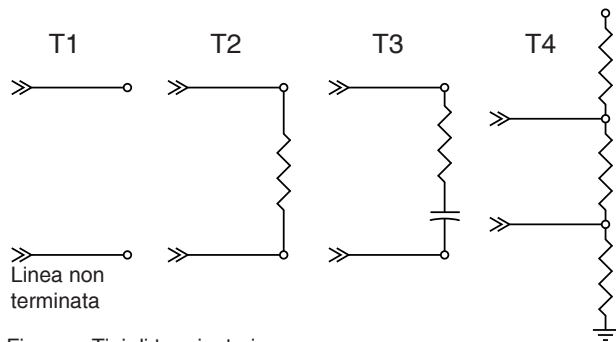
Fig.xxx : Tipi di terminatori
